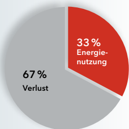
Herkömmliche Energieerzeugung
